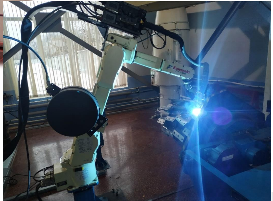
Сварка роботом по управляющей программе корпуса режущего барабана
