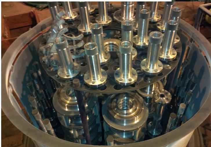
Установка загруженная деталями
